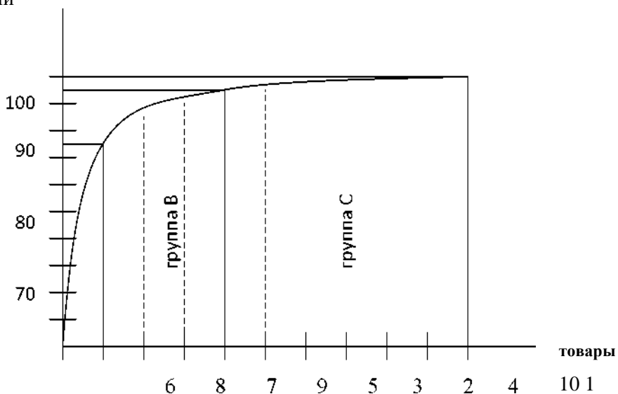
График сбыта по группам товаров (А, В, С)
