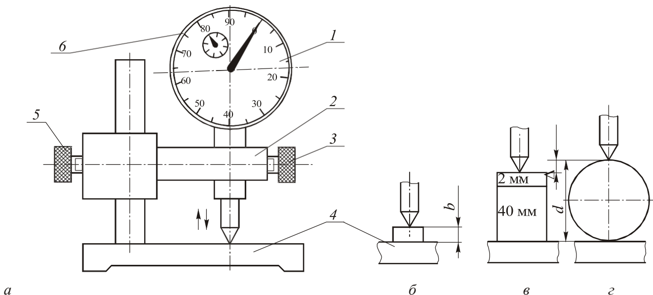
Рис.2. Измерение индикатором
