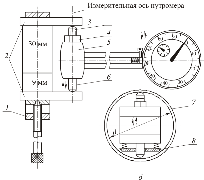
Рис.5. Индикаторный нутромер при настройке (а) (центрирующий мостик не показан) и при измерении (б)
