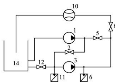
Рис. 1 Установка для испытания центробежных насосов:
